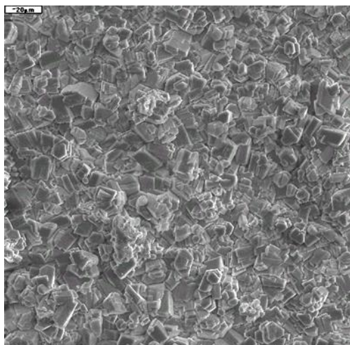
SURFACOTE MN 3, ingrandimento 500x
