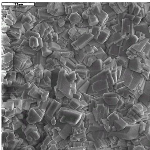
SURFACOTE MN 3, ingrandimento 1000x
